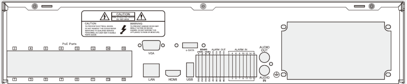
三十二路後背板示意圖
