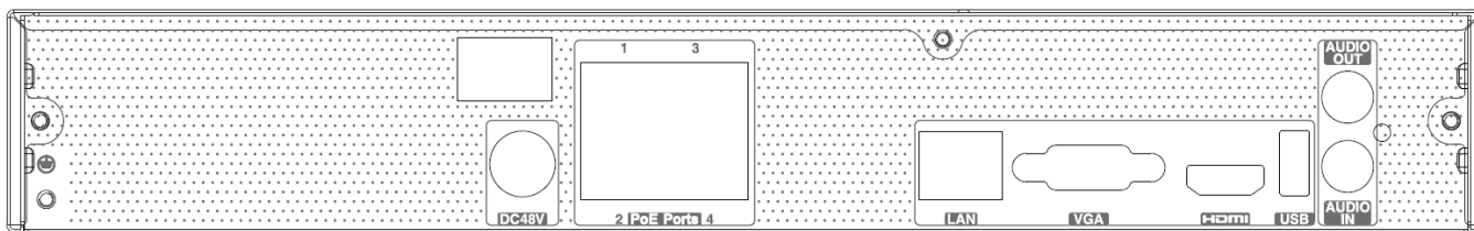
四路後背板示意圖
